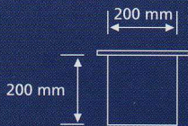
Mod. EMPOTRAR-2 (Molde de 7 m de largo)
