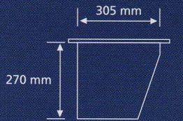
Mod. EMPOTRAR-4 (Molde de 6 m de largo)
