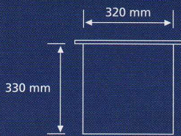
Mod. EMPOTRAR-1 (Molde de 7 m de largo)
