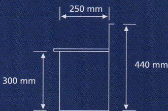
Mod. EMPOTRAR-6 (Molde de 6 m de largo)
